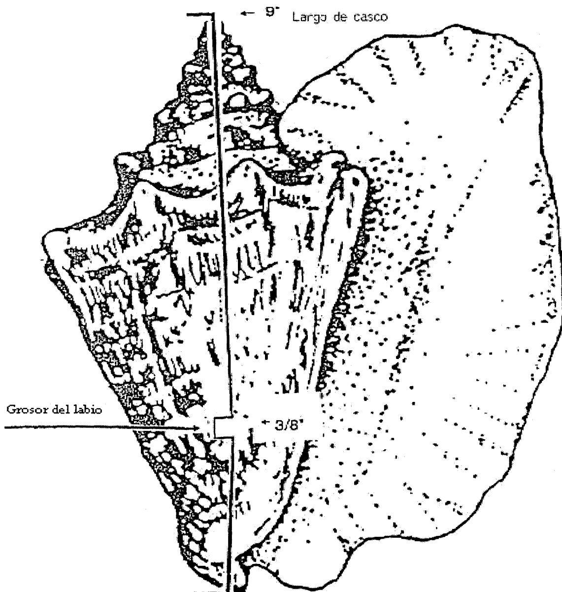
Figura 2 – Grosor del labio – una medida del borde de la concha del carrucho en aquel punto donde mayor sea su grosor
