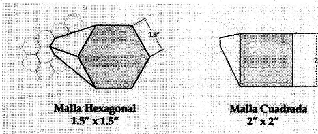
Figura 14. Apertura mínima de las mallas de alambre (rejillas)
