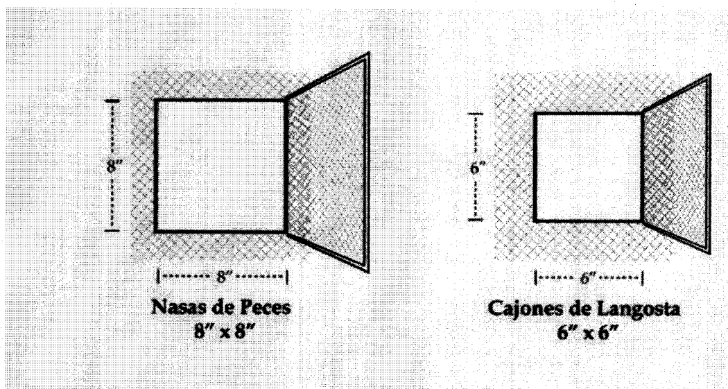
Figura 13. Apertura mínima del panel de escape de nasas
