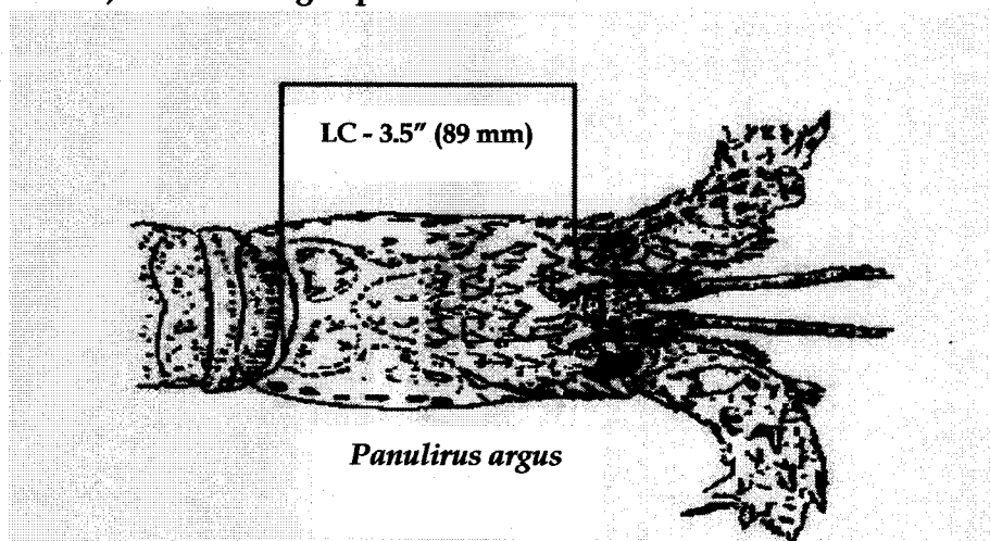
Figura 3. Largo de carapacho - LC - la medida de la cabeza de la langosta tomada en su comienzo desde la depresión orbital entre los cuernos de la langosta (surco de la proyección lateral) hasta el margen posterior del cefalotórax.
